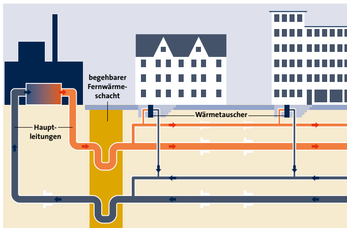
Schema Fernwärmeversorgung Quelle: Stadtwerke Bielefeld
